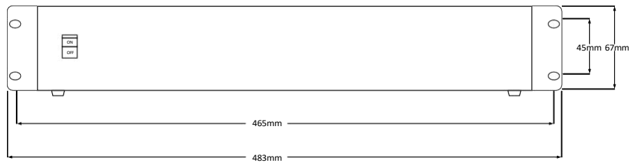
KS604前面板
