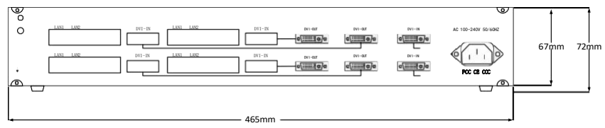
KS604后面板
