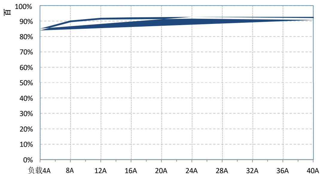
负载与效率曲线
