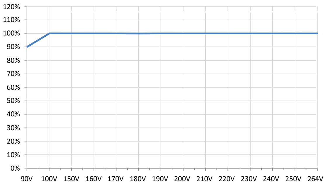
输入电压与负载关系曲线
