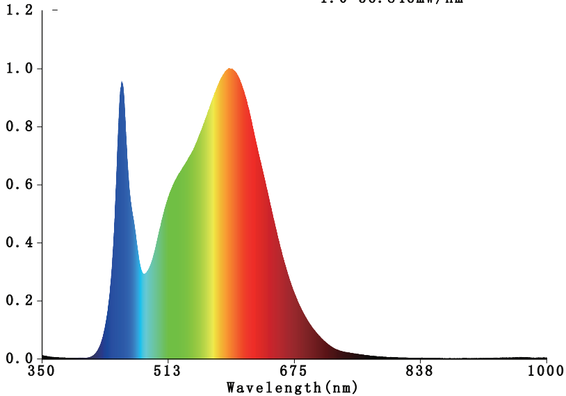
Spectrum 1.0=56.846mW/nm
