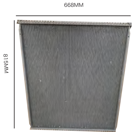
ZC-RAD-014 奔驰芯体 CORE BENZ ATEGO
