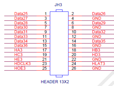
HEADER 13X2
