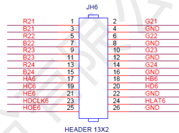
HEADER 13X2
