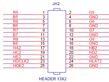
HEADER 13X2
