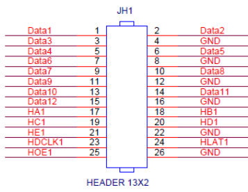
HEADER 13X2
