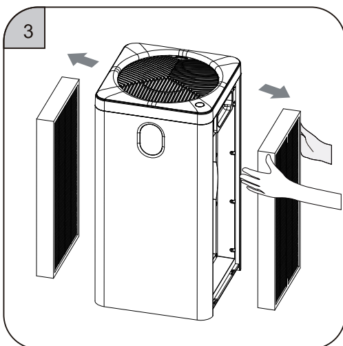
③ Retirez le nouvel écran de filtre avec un film plastique dans la machine.
