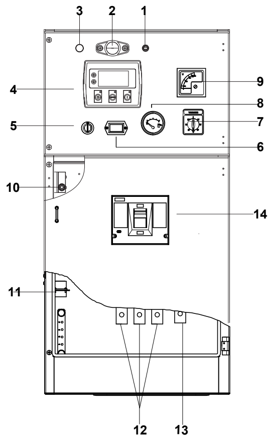
控制开关柜
