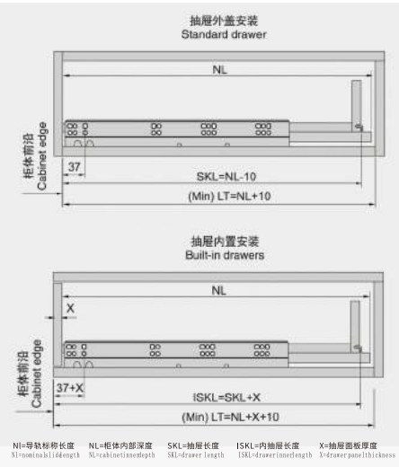
深度尺寸 Depth dimension
