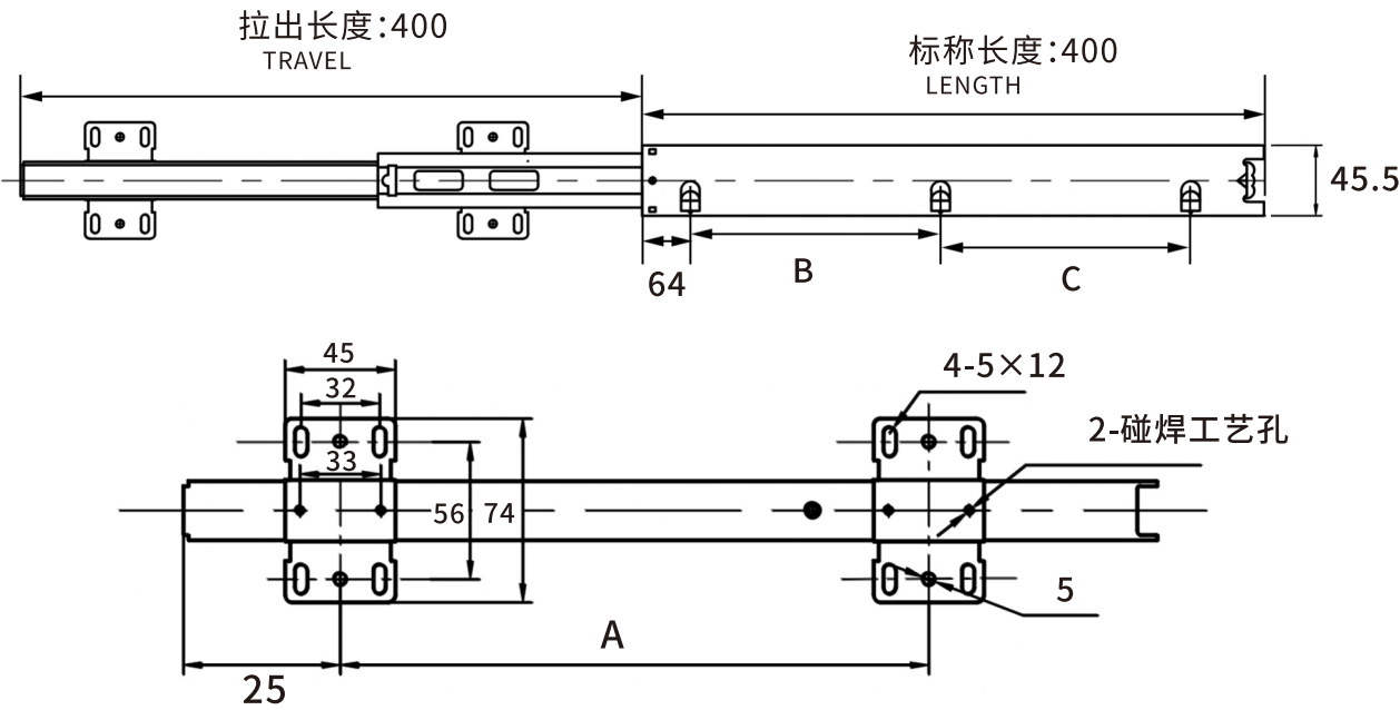
孔位示意图 Installation indication 图示Graphic:16"
