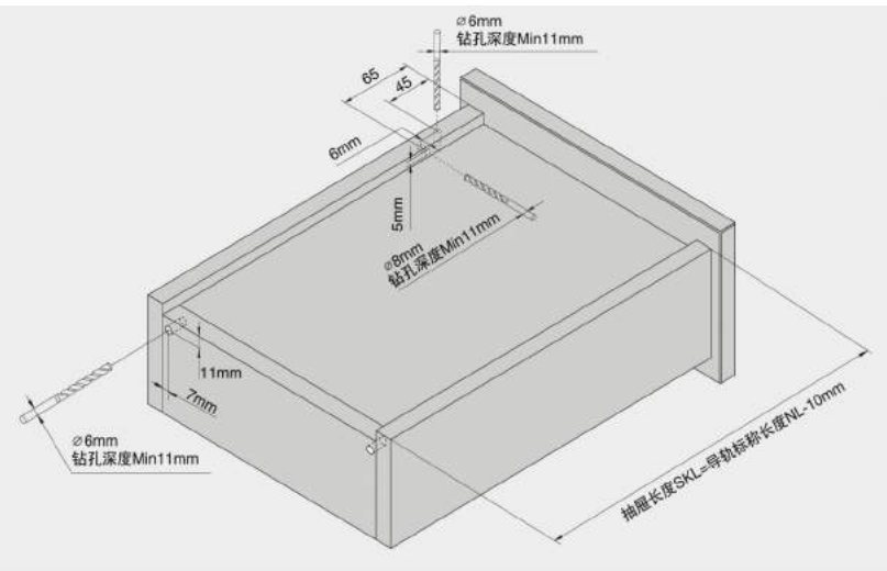
底部加工 Bottom processing
