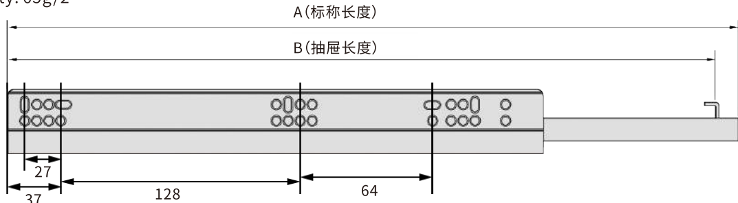
宽度尺寸 Width dimensions
