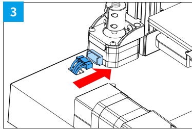
Z Motor 2 cable | Z-Motor 2 Kabel
