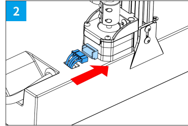
Z Motor 1 cable | Z-Motor 1 Kabel
