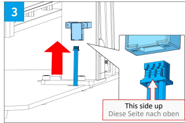
Z limit switch | Z-Endschalter
