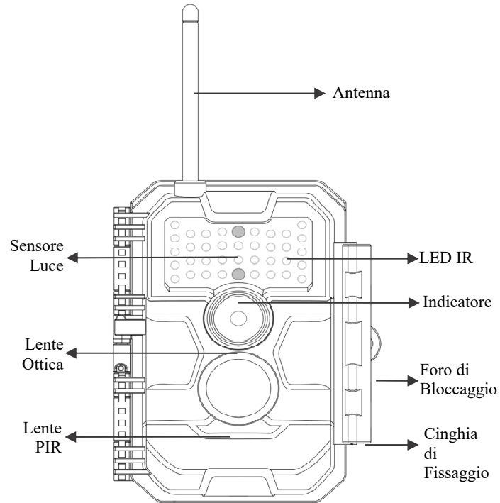
Figura 1: Visuale Frontale
