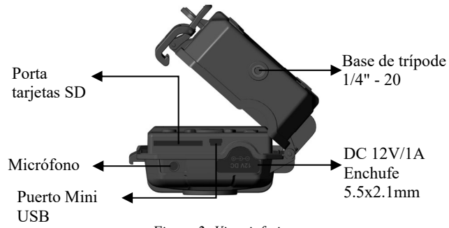
Figura 2: Vista inferior
