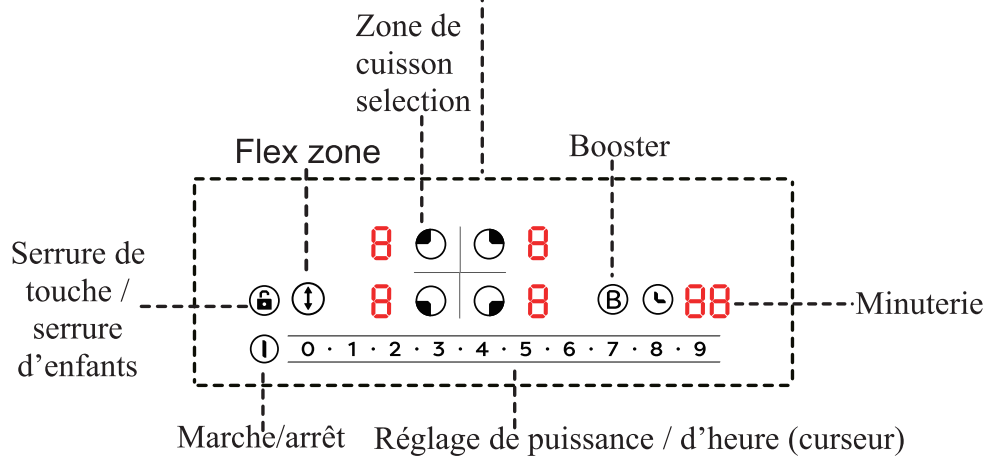
Panneau de commande
