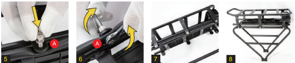
Figure 5,6 : Insérez la vis A et serrez Figure 7,8 : Installez les vis A des deux côtés tour à tour, et le porte-bagages est partiellement installé
