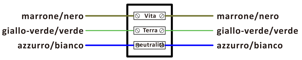
Bild. 3 Schema elettrico dell'inserto
