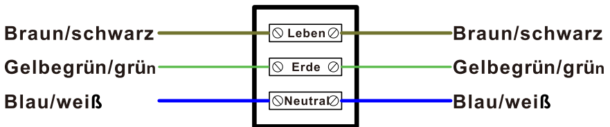
Bild. 3 Verdrahtungsplan vom Einlagung
