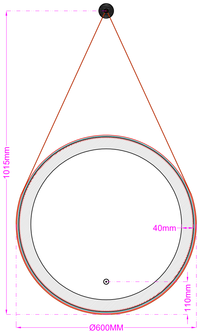
正面 GTBM09-6060
