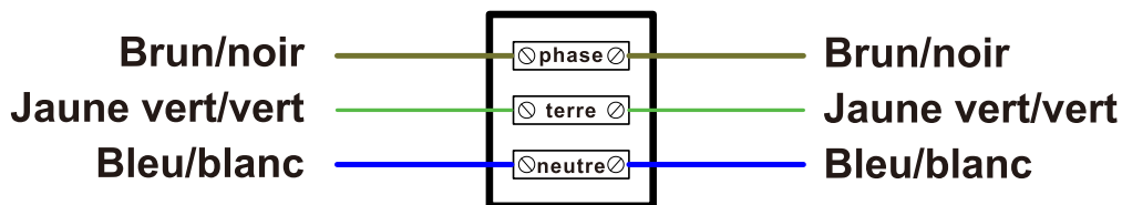
Bild. 3 Schéma de câblage des bornes d'entrée
