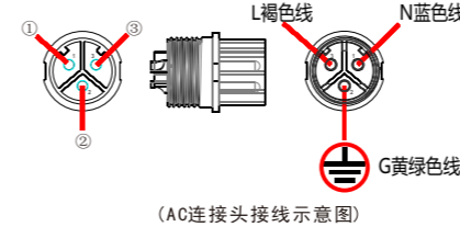
(AC连接头接线示意图)
